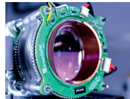
Blick unter das Gehäuse: Der Unterwasser-Laserscanner ULi taucht bis zu 300 Meter tief.
